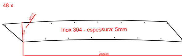
Dimensões - Chapa de aço inoxidável 304 Escala 1/3
